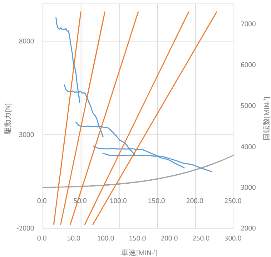
BONGO MANBOW T/C 走行性能曲線
